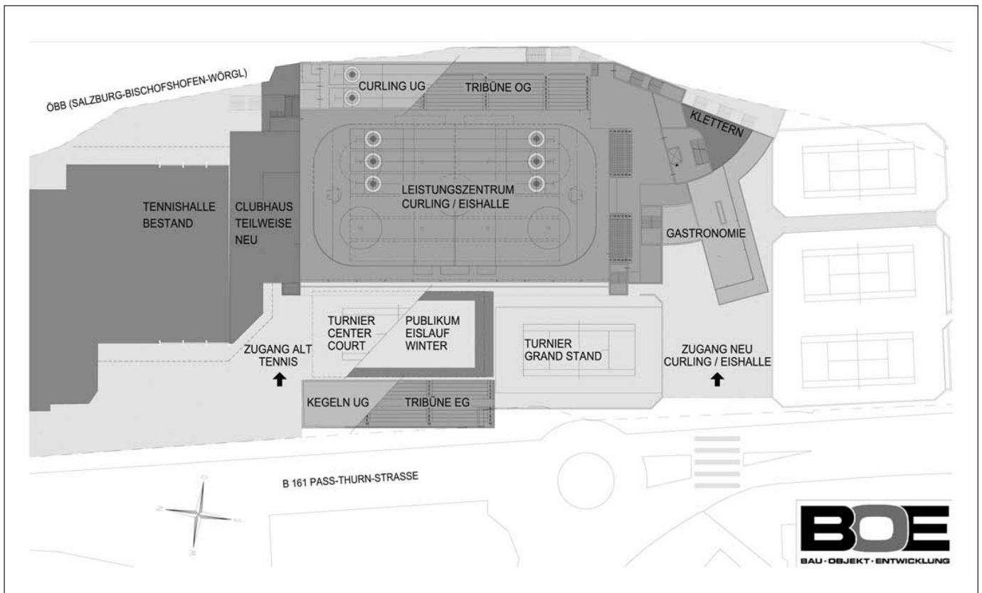
Vorläufige planliche Übersicht Mehrzwecksportanlage Kaps, Stand 15. 3. 2005.
